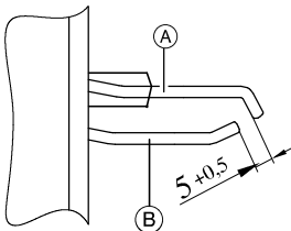
Vue latérale
